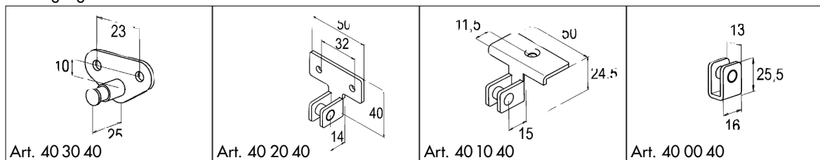
Befestigungselemente unten
