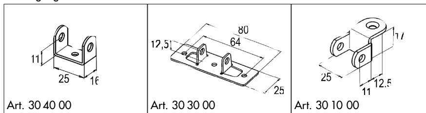
Befestigungselemente unten
