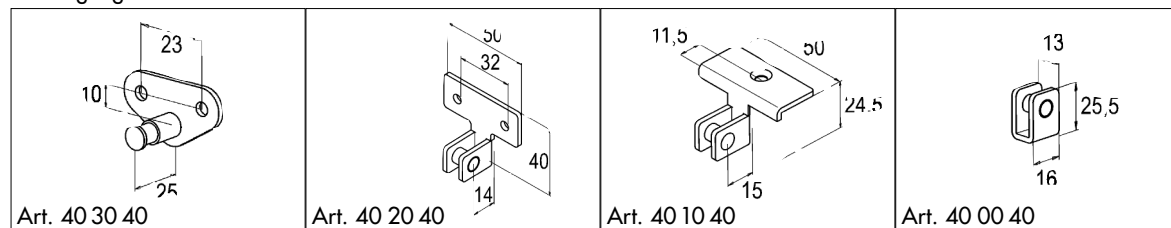
Befestigungselemente unten
